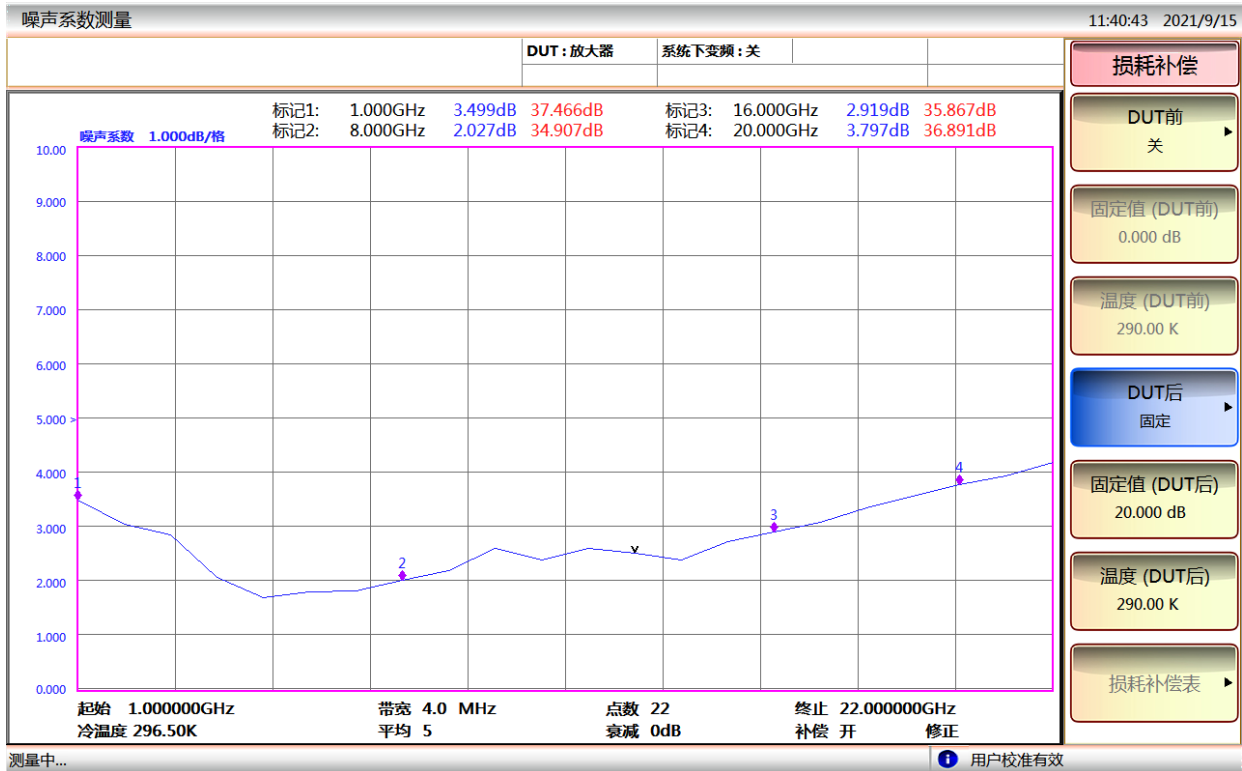
NF Test 1-22GHz
